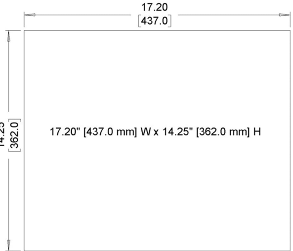
Cutout Dimensions
