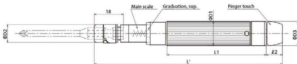
BMRD15CN2, 30CN2
