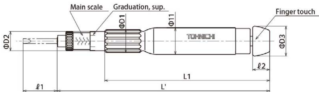
AMRD 1CN~8CN
