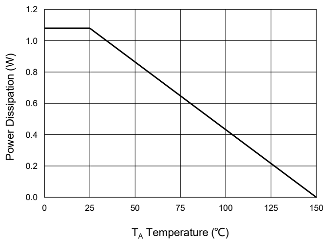
Fig. 11 - P D Dissipation
