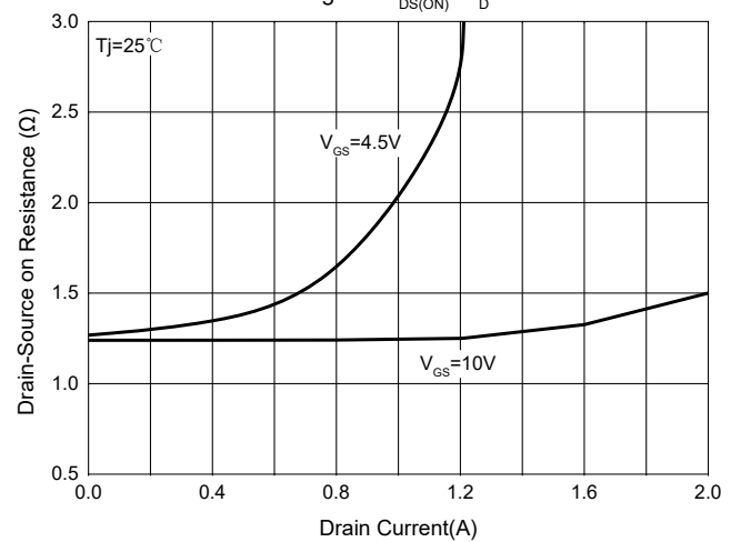
Fig. 4 - R_{DS(ON)} -- I_D
